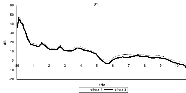
Figura 2. Espectros de longo termo (ELT) de duas leituras de S1
