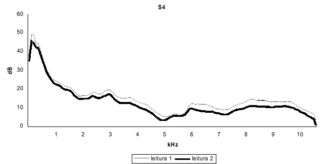
Figura 5. Espectros de longo de termo (ELT) de duas leituras de S4
