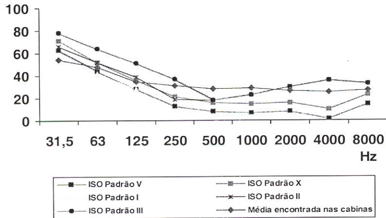
Figura 2 – Comparação entre valores médios (em dB), por freqüência (Hz), mensurados nas cabinas e o Padrão V da Norma ISO 8253-1
